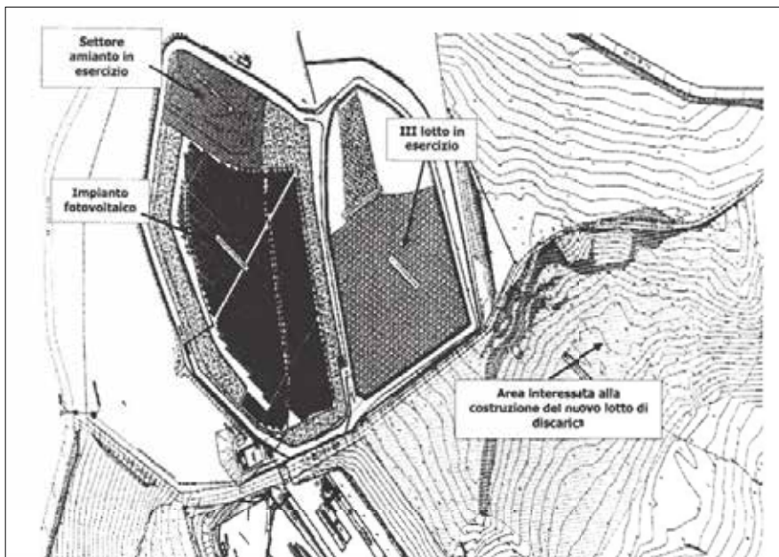
Un particolare del progetto di ampliamento tratto dalla delibera della Regione Basilicata
