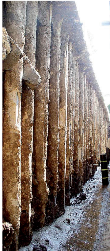
PARATIA Al centro della perizia la misurazione della lunghezza di una serie di micropali per un muro di sostegno
